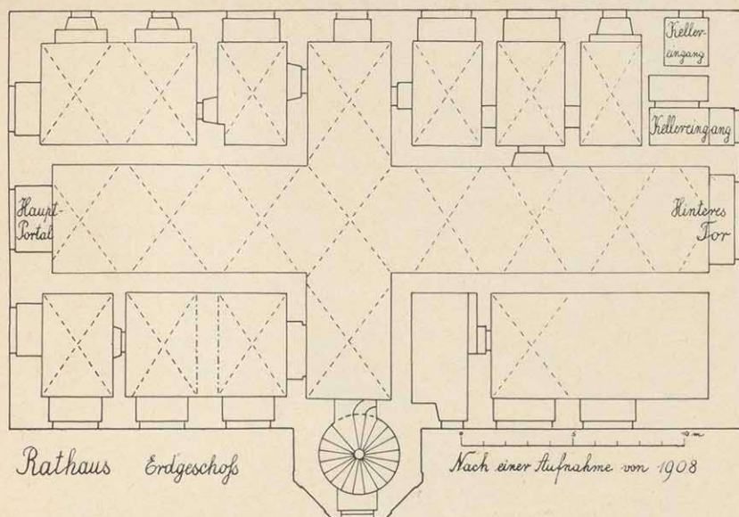
Grundriß des Erdgeschoßes
