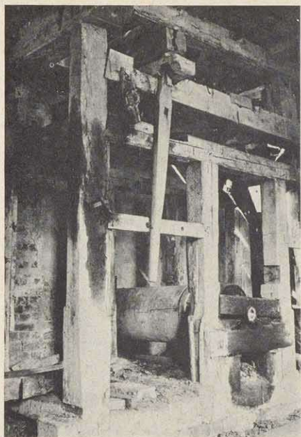
Das waren die traurigen Reste der Märlmühle in Oberlauter, die inzwischen im Natur-Museum zu einer originalgetreuen Anlage ergänzt wurden.
