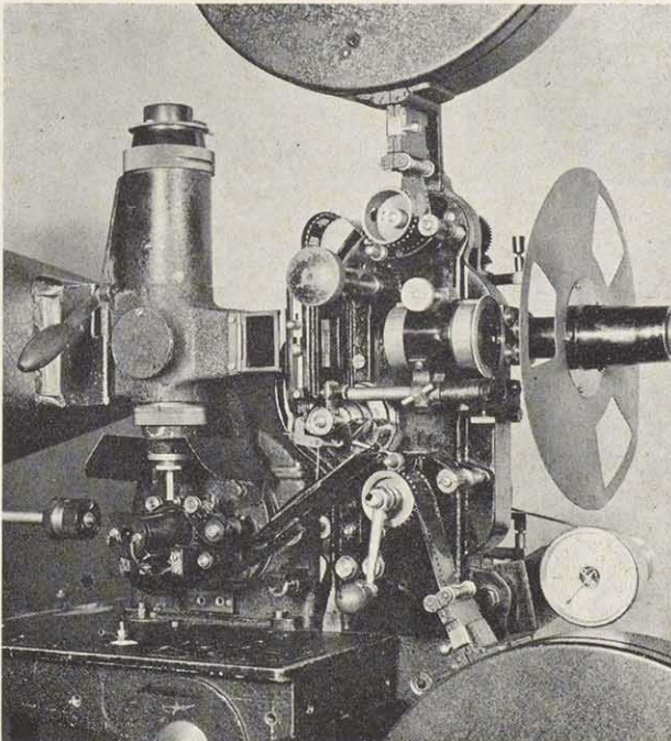
Triegon Tonfilm- Wiedergabe, Apparat von Vogt, Engl und Massole, 1923
