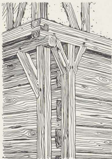
Eckkonstruktion am Umgebindehaus in Nentschau
