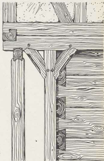
Ansicht der Eckkonstruktion (Giebelseite)
