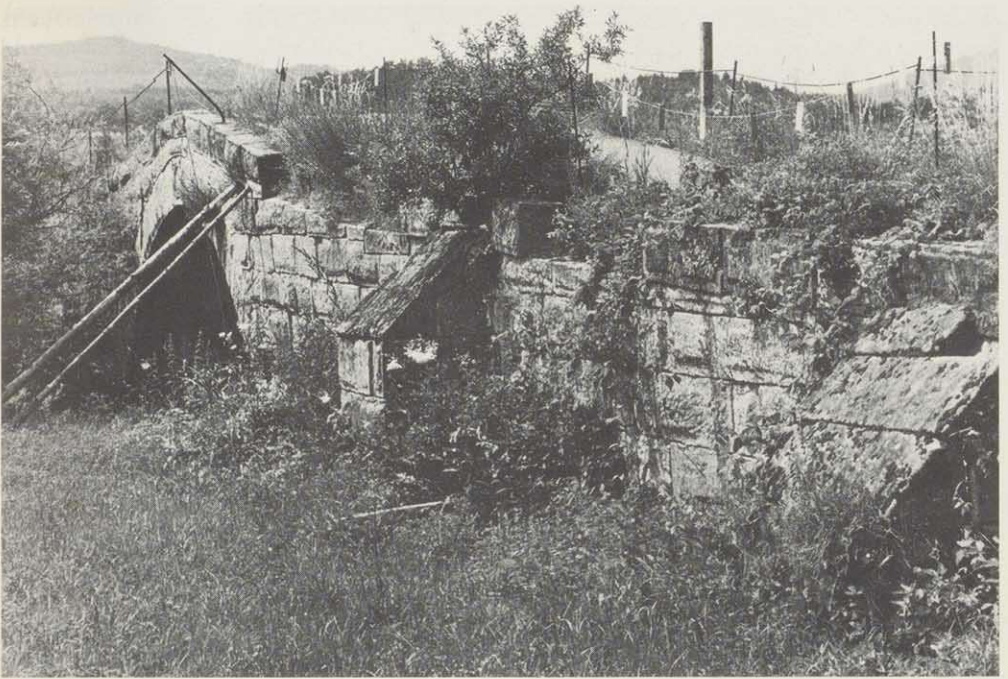
Leucherhofbrücke über die Baunach: Sommer 1979 — abgestützt — Geländer fehlt — auf 3,5 Tonnen beschränkt — die Flügelmauern drohen einzustürzen
