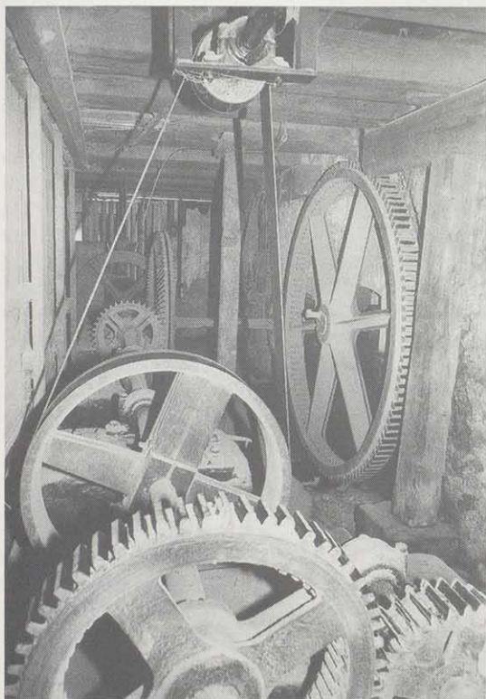
Nankendorfer Mühle 1990 Transmission zum Erhöhen der Drehzahl zwischen Wasserrad (re.) und Arbeits- maschinen
