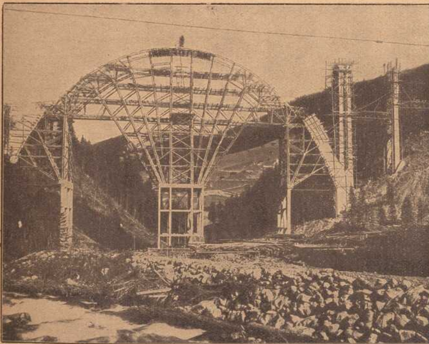
Vom Bau der elektrischen Chur-Arosa-Bahn: Die Bogenbrücke aus Eisenbeton bei Langwies.
