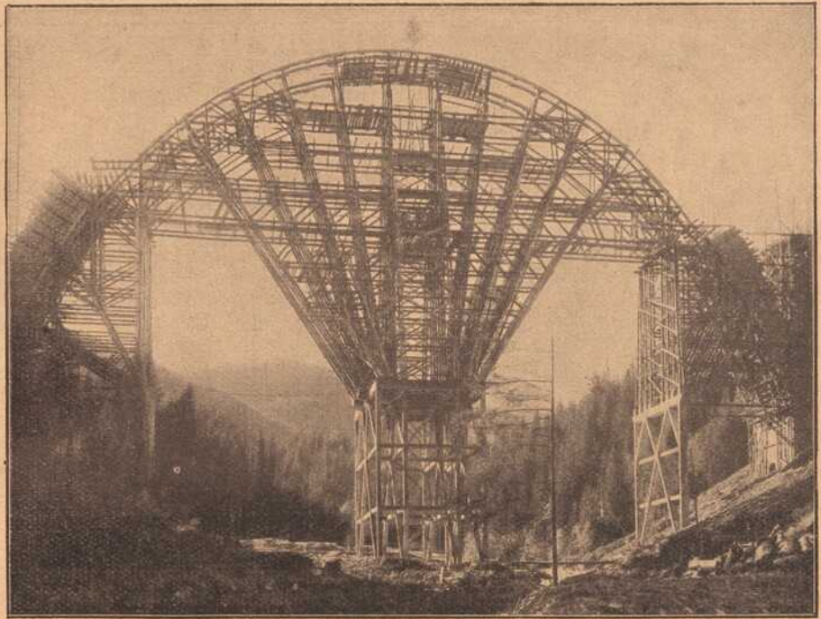
Vom Bau der Chur-Arosa-Bahn: Das Leegerüst zum Bogenviadukt bei Langwies. Derselbe wird die größte Bogenbrücke aus Eisenbeton, die bisher hergestellt worden ist. Spannweite des Bogens 100 Meter.
