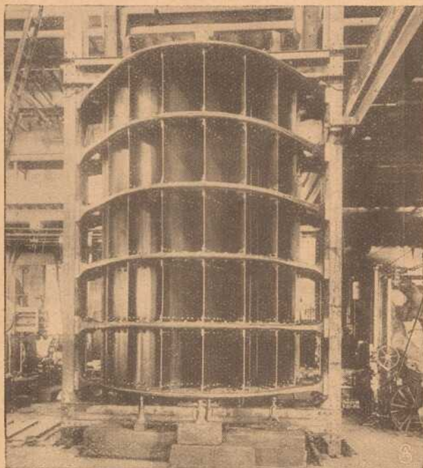
Eine Riesenturbine in Brighton Beach, die von der Meeresströmung getrieben wird.
